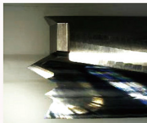
ウレタンゴム加工のために開発された独自の刃形状
