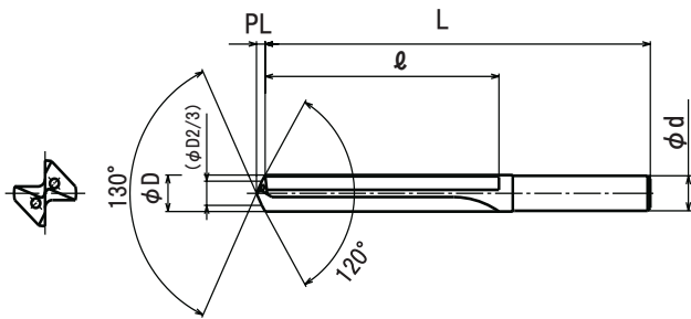
φD公差
