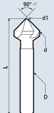
90° コバルトハイス鋼 + TiN
